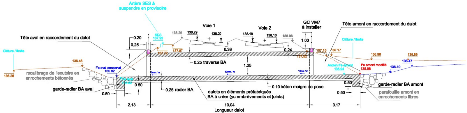
Figure 10 : vue en coupe longitudinale de l'ouvrage hydraulique envisagé au PK 714 – source : SNCF
